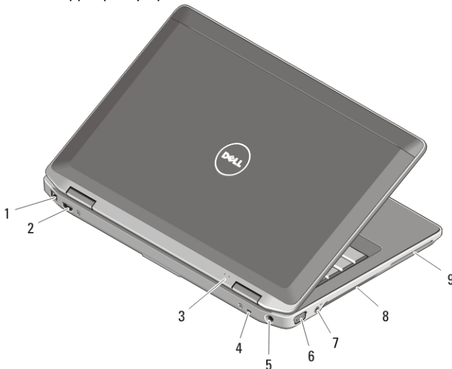
Figur 2: Sett bakfra
